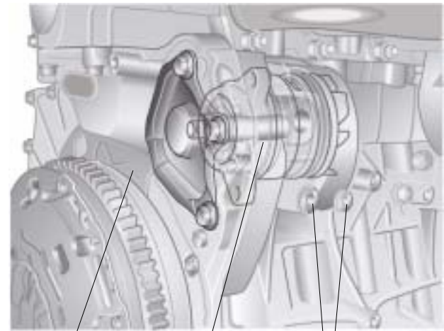
305_049 Steuergehäuse Kühlmittelpumpe Kühlmittelablassschraube
